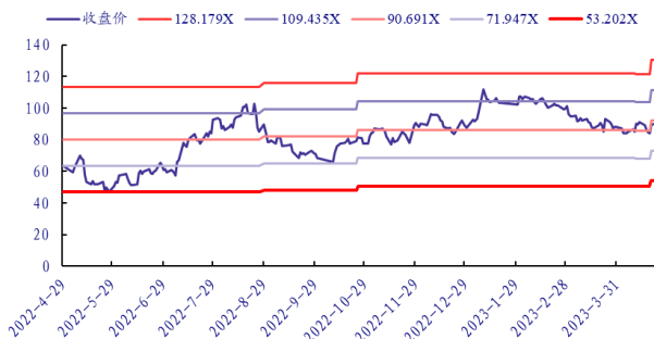
图 5：PE-Bands
