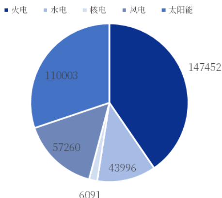
图13: 2025 年上半年全国电源装机结构 (万千瓦)
