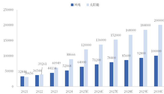
图39: 新能源累计装机预测（万千瓦）
