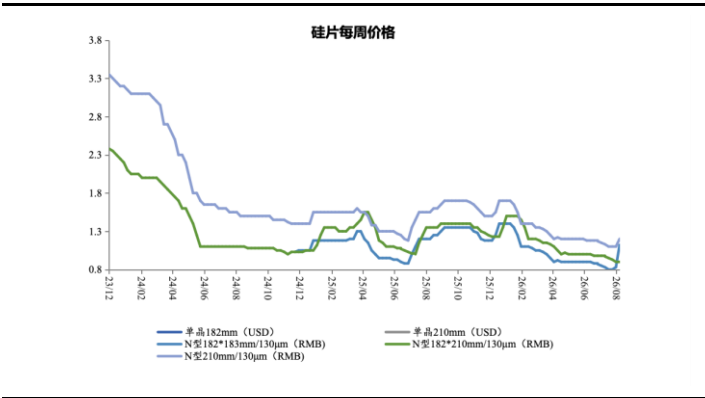
图31：硅片价格走势（元/片）
