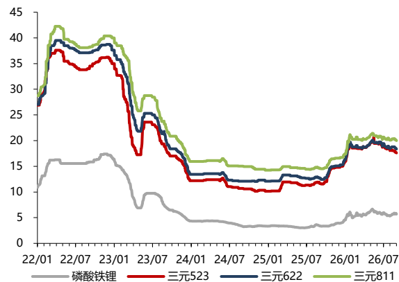
图18: 部分电池正极材料价格走势 (万元/吨)
