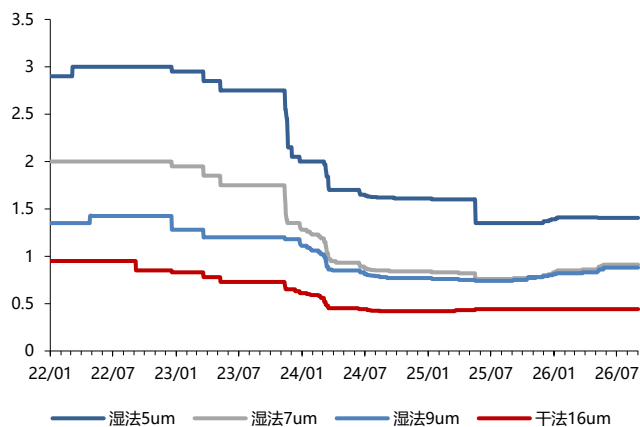
图20: 部分隔膜价格走势 (元/平方米)
