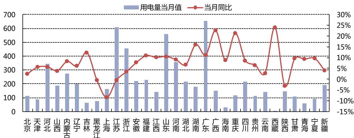
图表 24 7月用电量分区域情况 (单位: 亿千瓦时)
