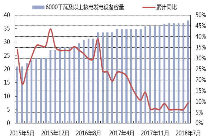
图表 27 核电发电设备容量情况 (单位: 百万千瓦)
