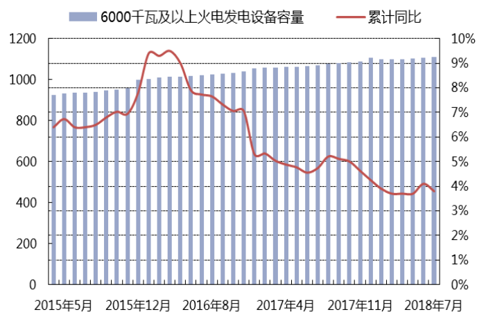
图表 25 火电发电设备容量情况 (单位: 百万千瓦)
