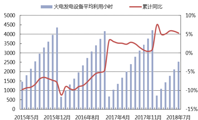
图表 29 火电发电设备平均利用小时
