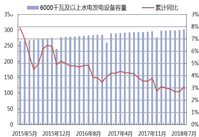
图表 26 水电发电设备容量情况 (单位: 百万千瓦)
