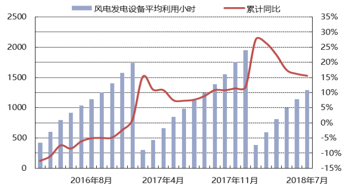
图表 32 风电发电设备平均利用小时
