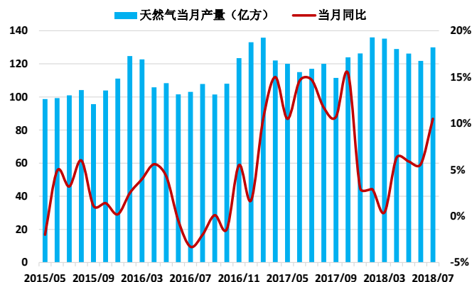
图表 39 天然气月度生产量 (单位: 亿方)
