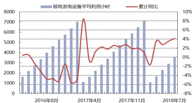
图表 31 核电发电设备平均利用小时
