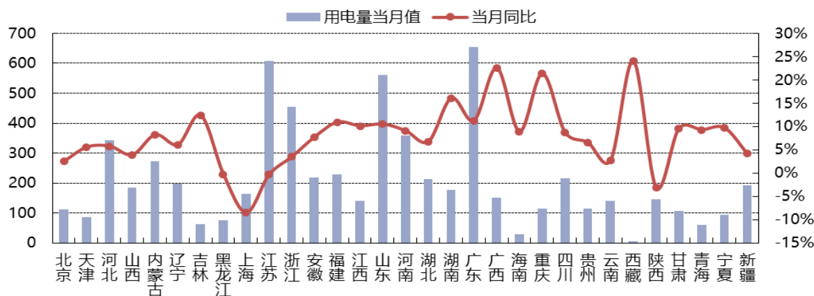
图表 24 7月用电量分区域情况 (单位: 亿千瓦时)
