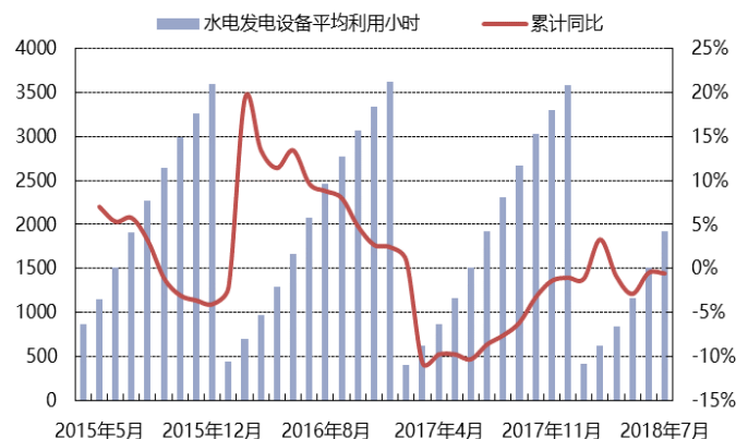
图表 30 水电发电设备平均利用小时
