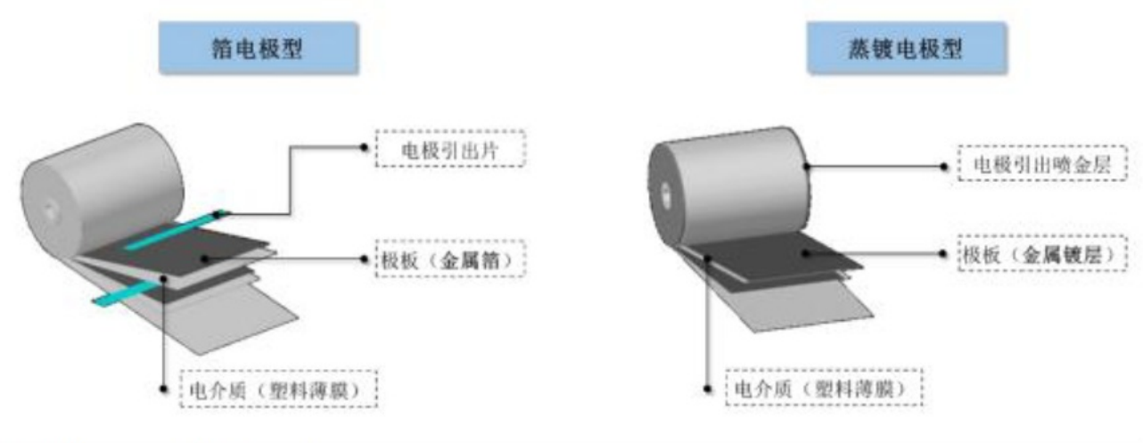
图13: 两种典型的薄膜电容器排列结构
