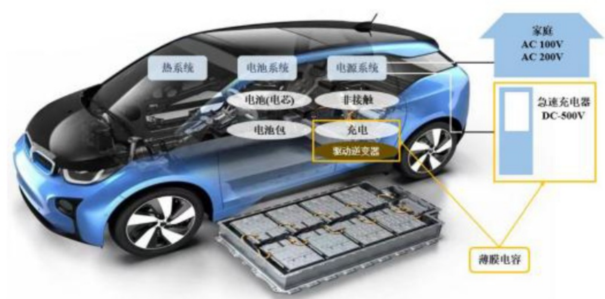
图22: 薄膜电容器在新能源汽车电驱上的应用
