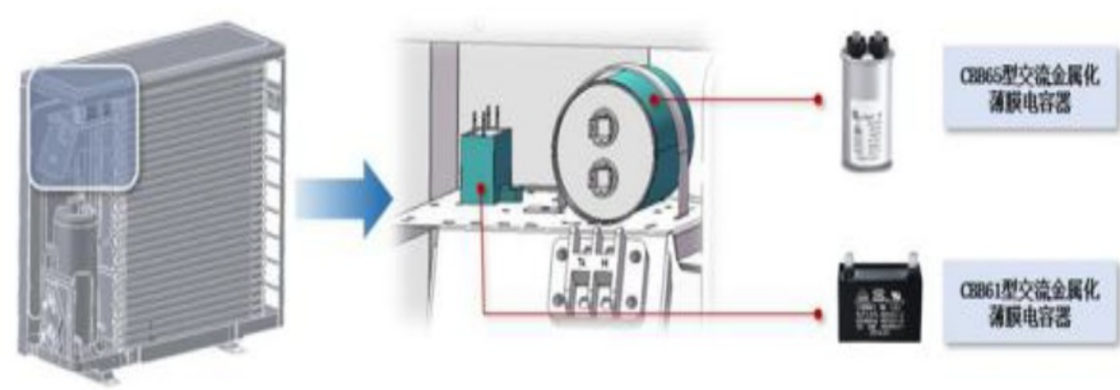
图7：电机电容器在空调外机的具体应用
