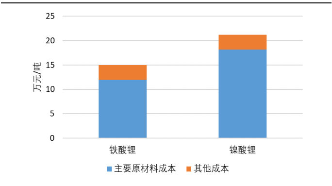
图表 11：典型正极补锂剂成本测算
