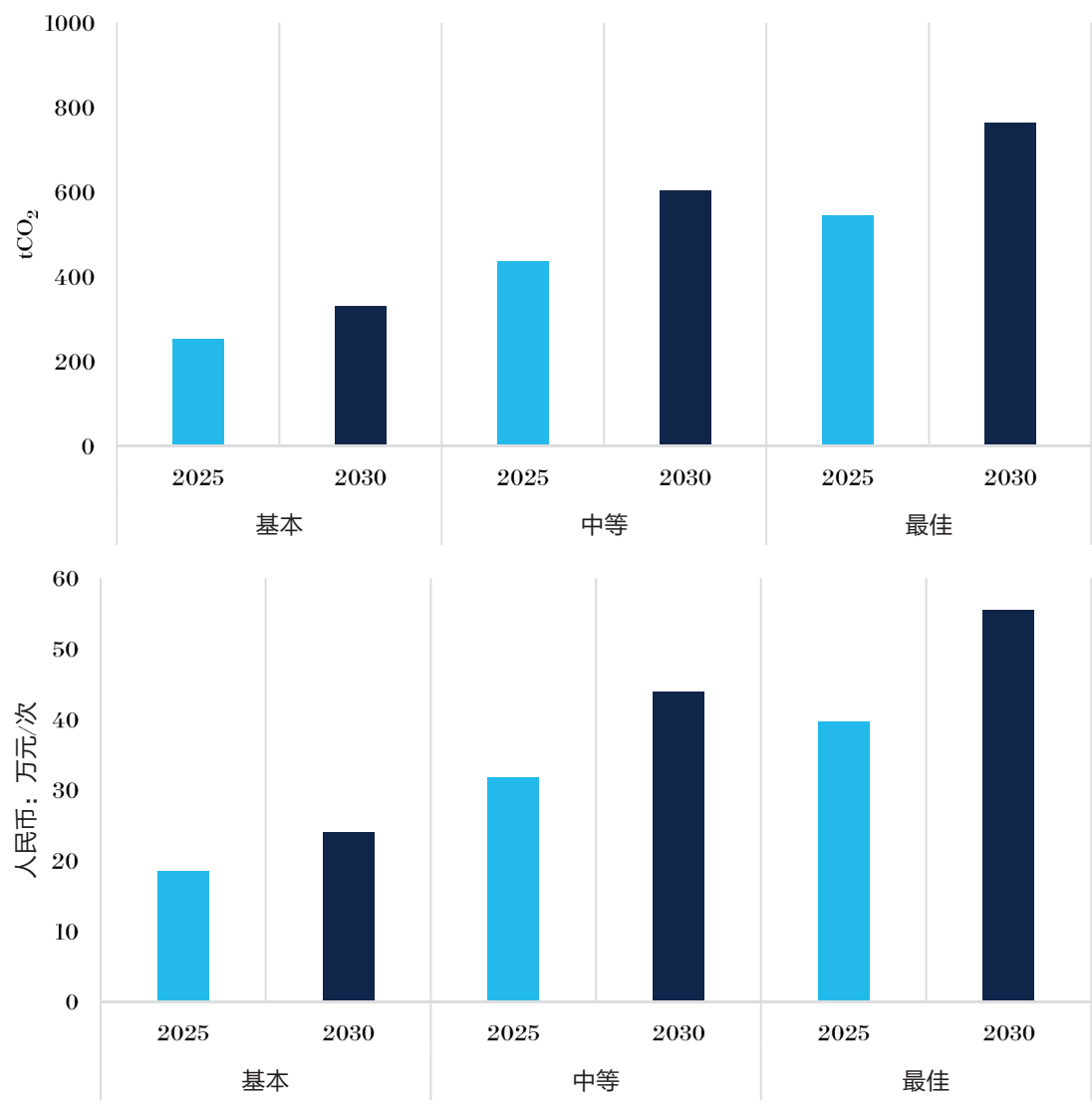
图 4-11 2025-2030 年深圳市电动汽车响应二氧化碳经济效益
