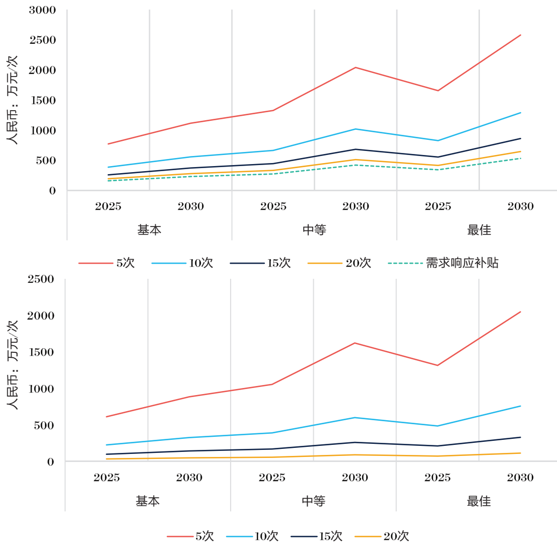
图 4-9 2025-2030 年深圳市电动汽车响应可避免发电成本和净经济收益
