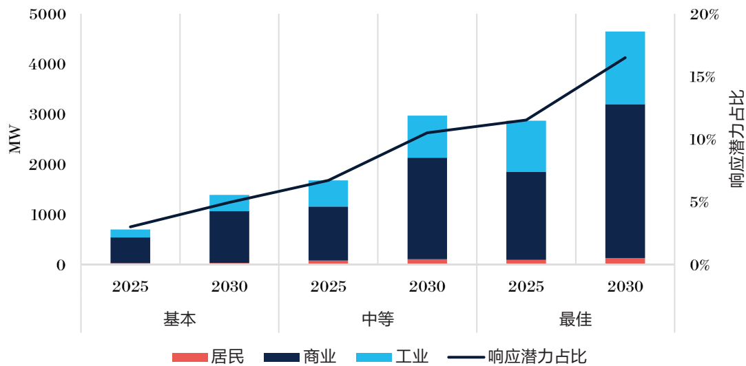
图 4-2 2025-2030 年深圳市空调响应潜力
