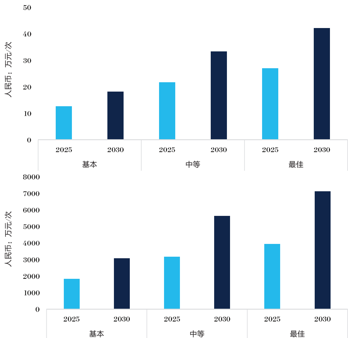
图 4-10 2025-2030 年深圳市电动汽车经济性评估
