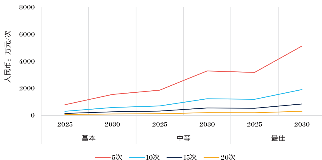
图 4-6 2025-2030 年深圳市空调响应可避免发电成本和净经济收益
