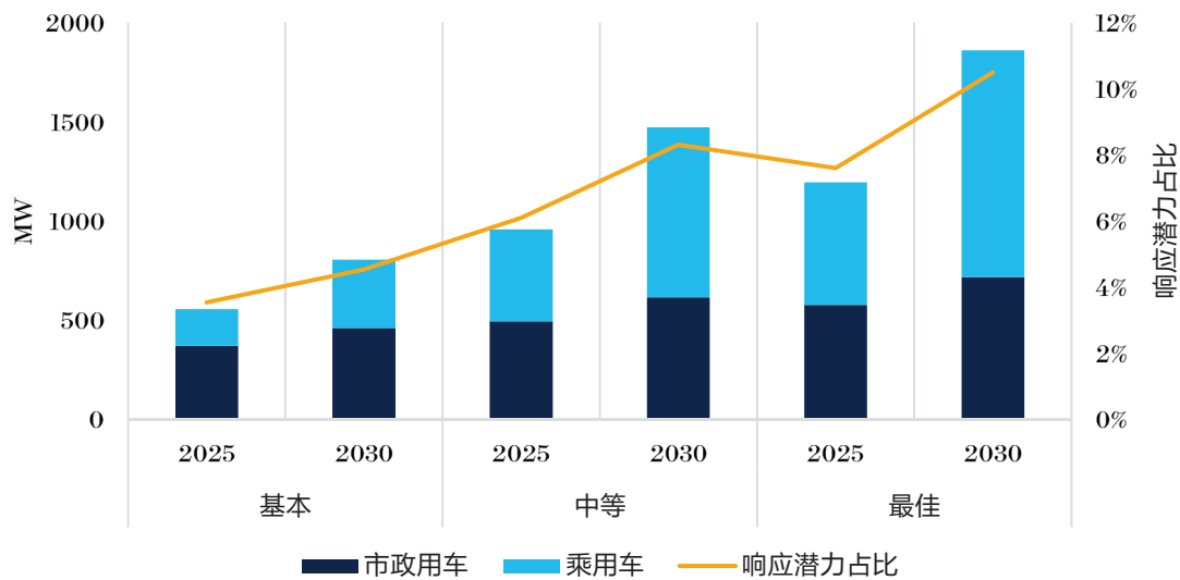
图 4-4 2025-2030 年电动汽车响应潜力
