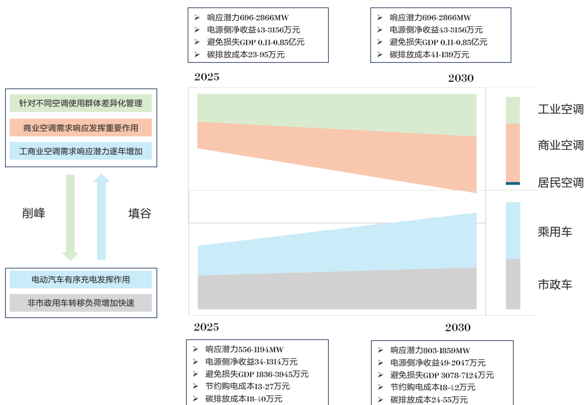
图 5-1 深圳市响应潜力评估结果
