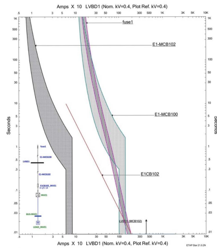
图9 不同断路器和熔断器的匹配
