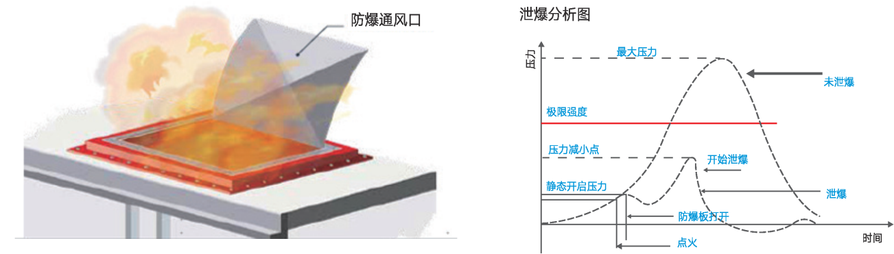
图20 泄爆示意图
