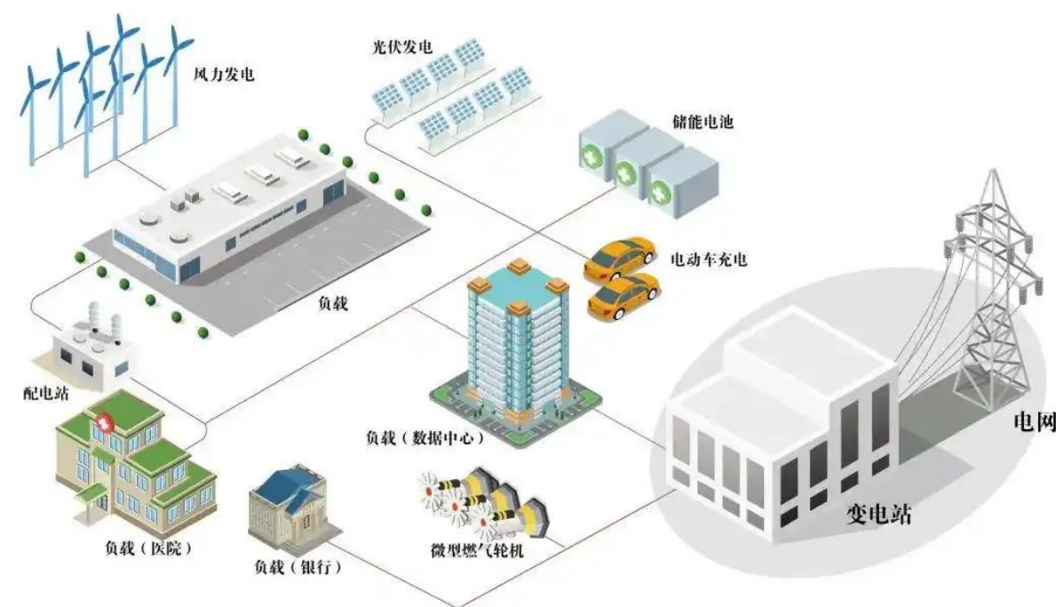
图 1：微电网示意图
