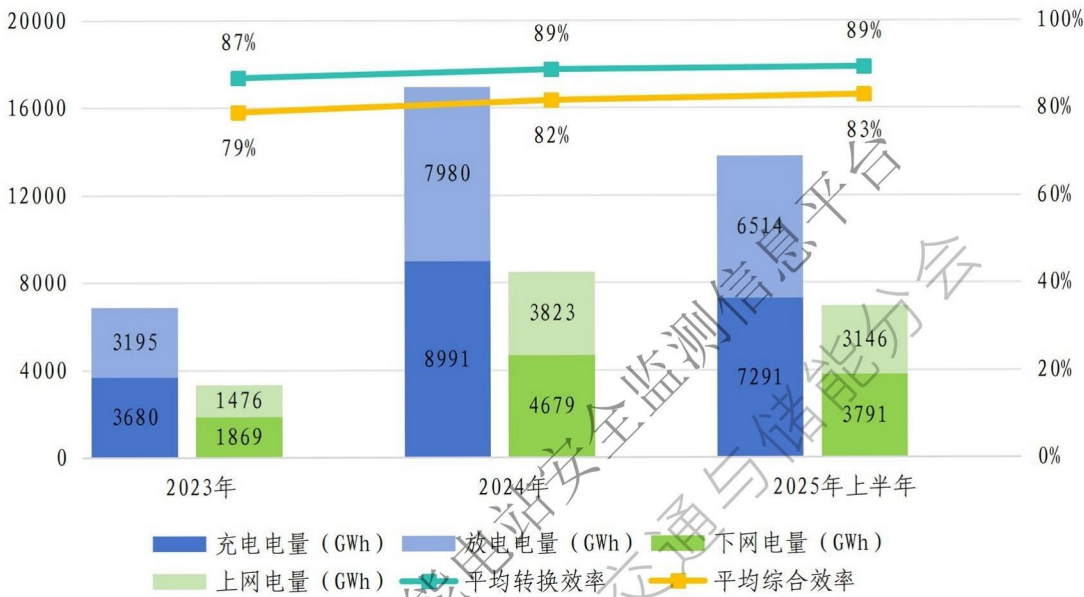
图 3-1 近 3 年电化学储能能效情况
