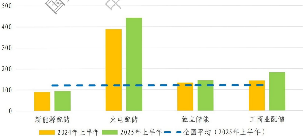
图 2-2 典型应用场景下电化学储能平均等效充放电次数
