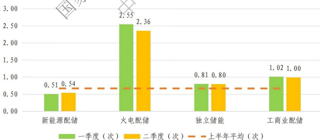
图 2-5 典型应用场景下电化学储能各季度日均等效充放电次数
