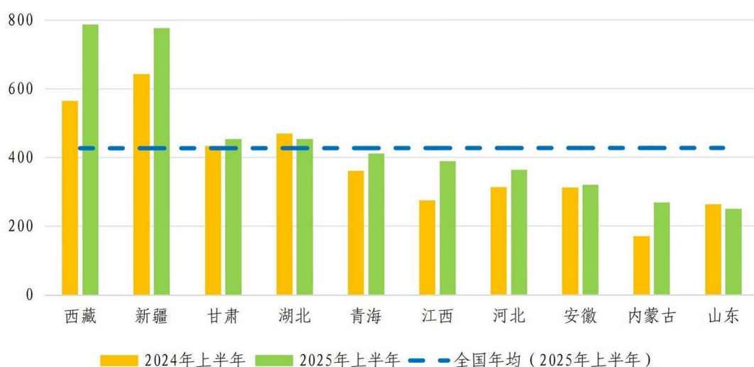
图 2-7 典型区域新能源配储平均利用小时数
