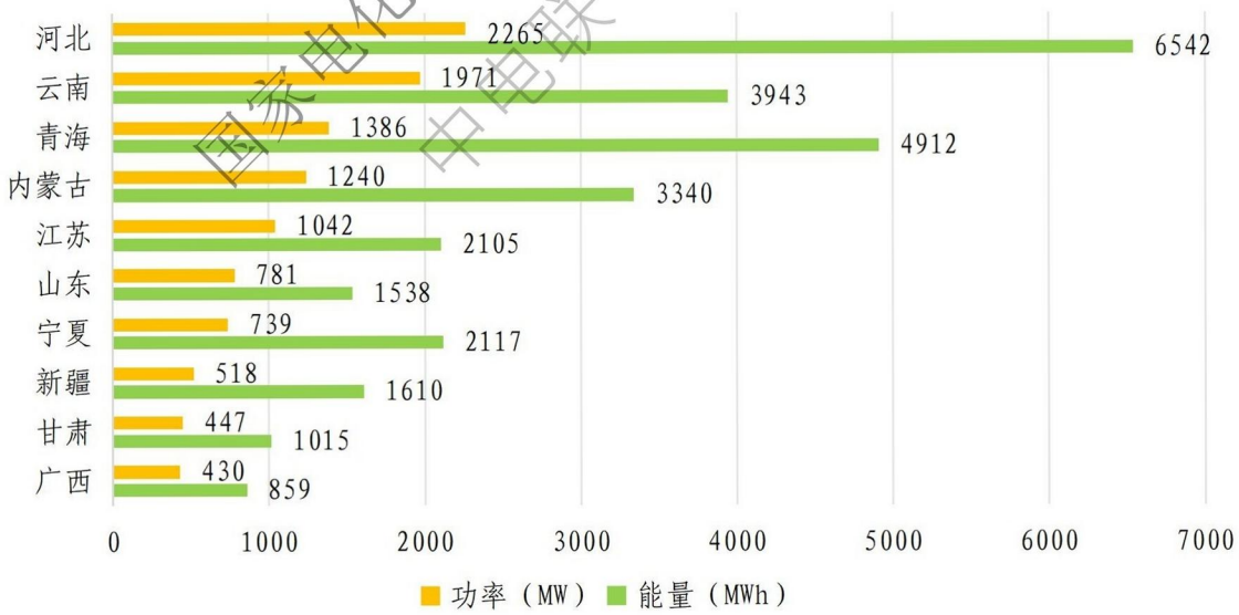
图 1-6 电化学储能电站新增总装机排名前十的省份
