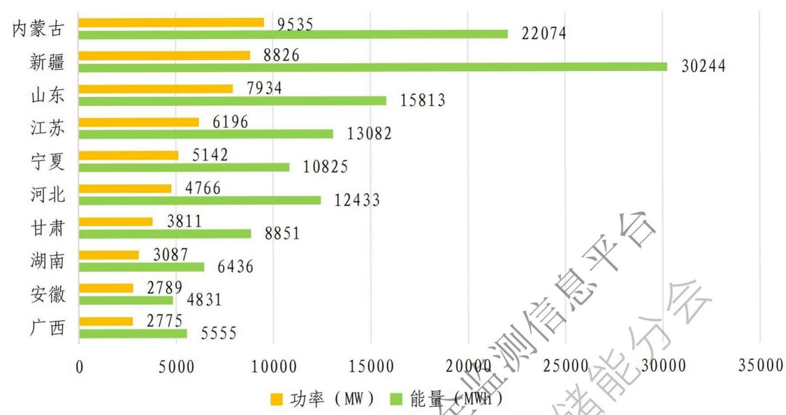
图 1-7 电化学储能电站累计总装机排名前十的省份
