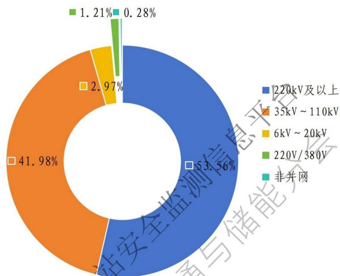
图 1-9 电化学储能电站接网电压等级分布情况
