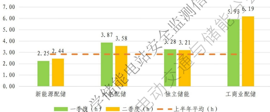
图 2-4 典型应用场景下电化学储能各季度日均利用小时数
