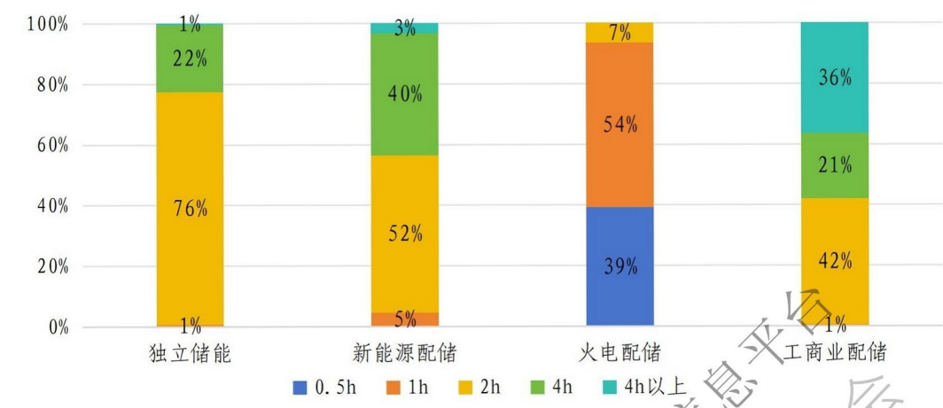
图 1-5 电化学储能典型应用场景储能时长分布情况
