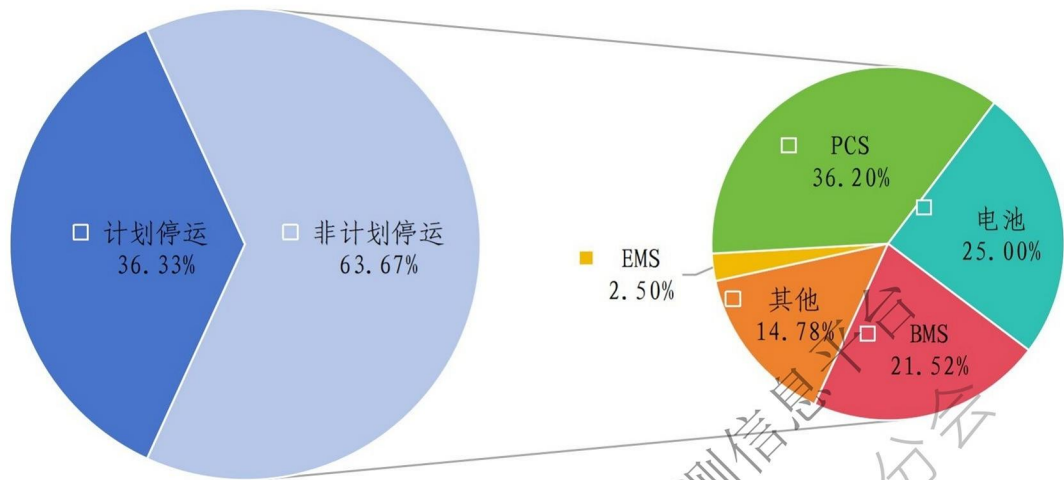
图 4-1 2025 年上半年电化学储能停运次数分布情况
