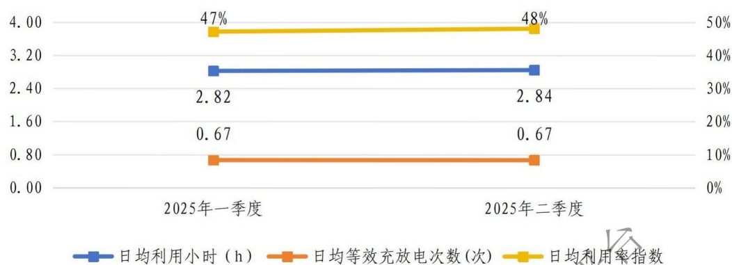
图 2-3 2025 年电化学储能季度运行情况
