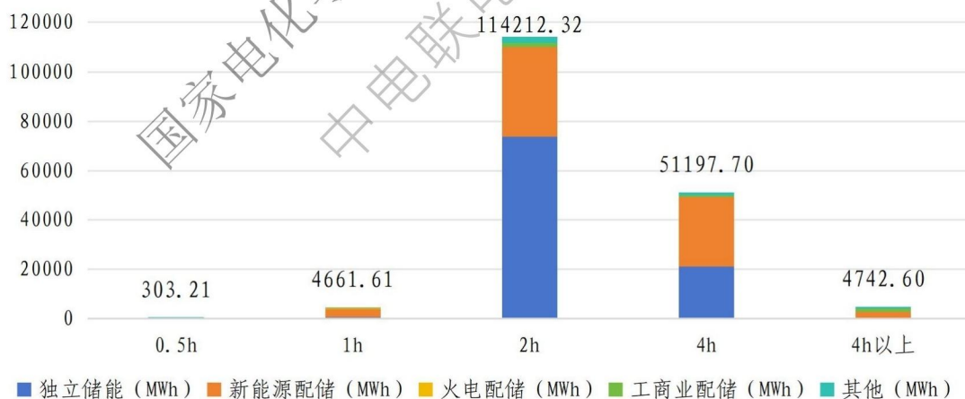
图 1-4 电化学储能储能时长分布情况
