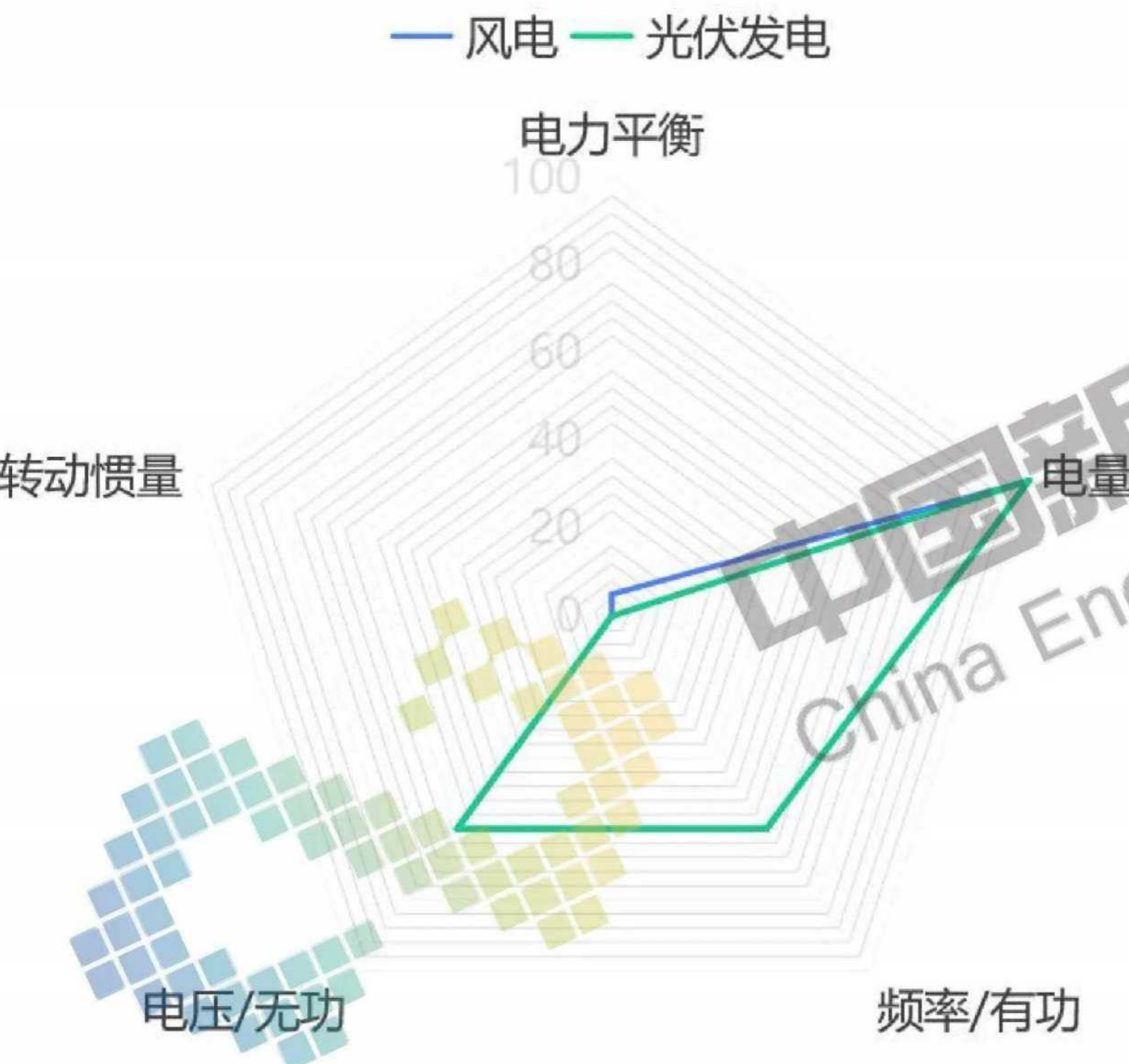
风电光伏发电出力特性图
