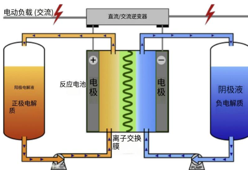
图 17：液流电池工作原理示意图
