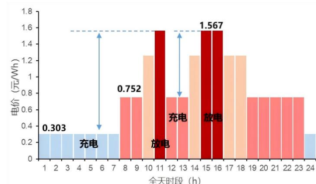
图 10：一个峰谷差和一个峰平差：两充两放
