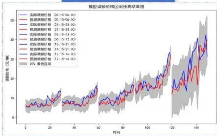
模型调频价格区间预测结果图
