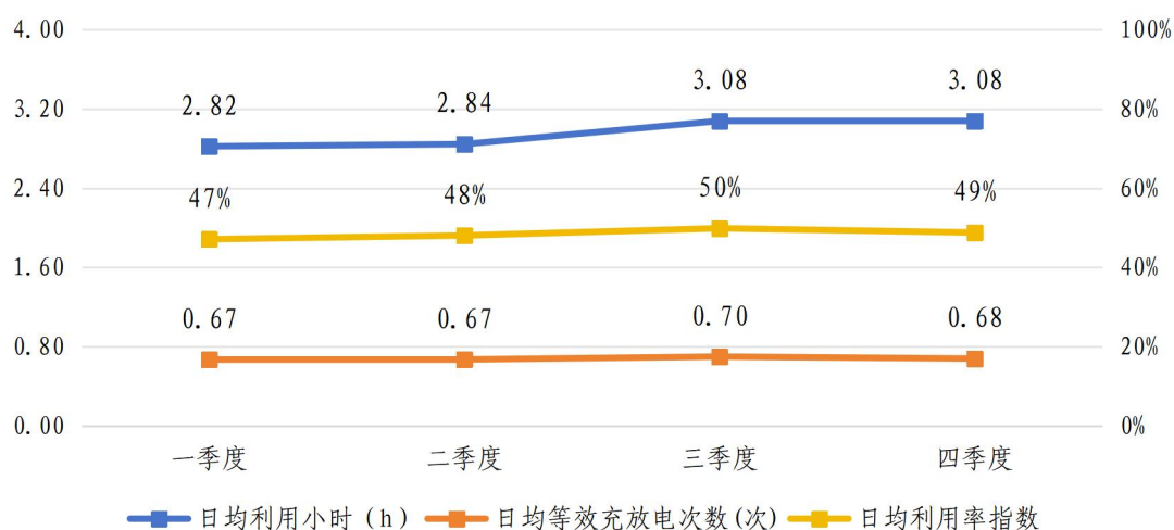
图 2-3 2025 年电化学储能季度运行情况
