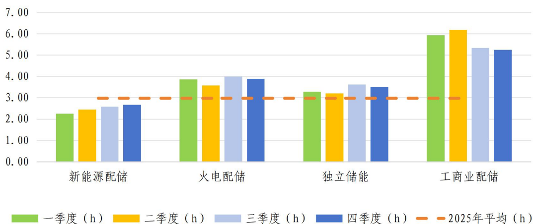
图 2-4 典型应用场景下电化学储能各季度日均利用小时数
