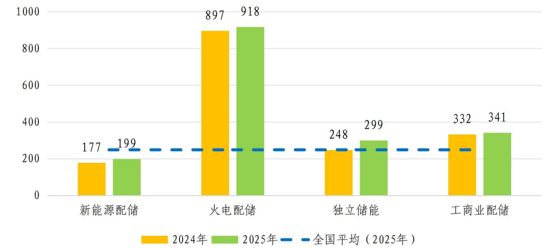
图 2-1 典型应用场景下电化学储能年均利用小时数
