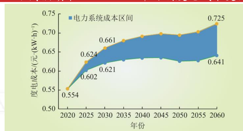
图表16：不同预期下2020—2060年终端度电成本变化情况
