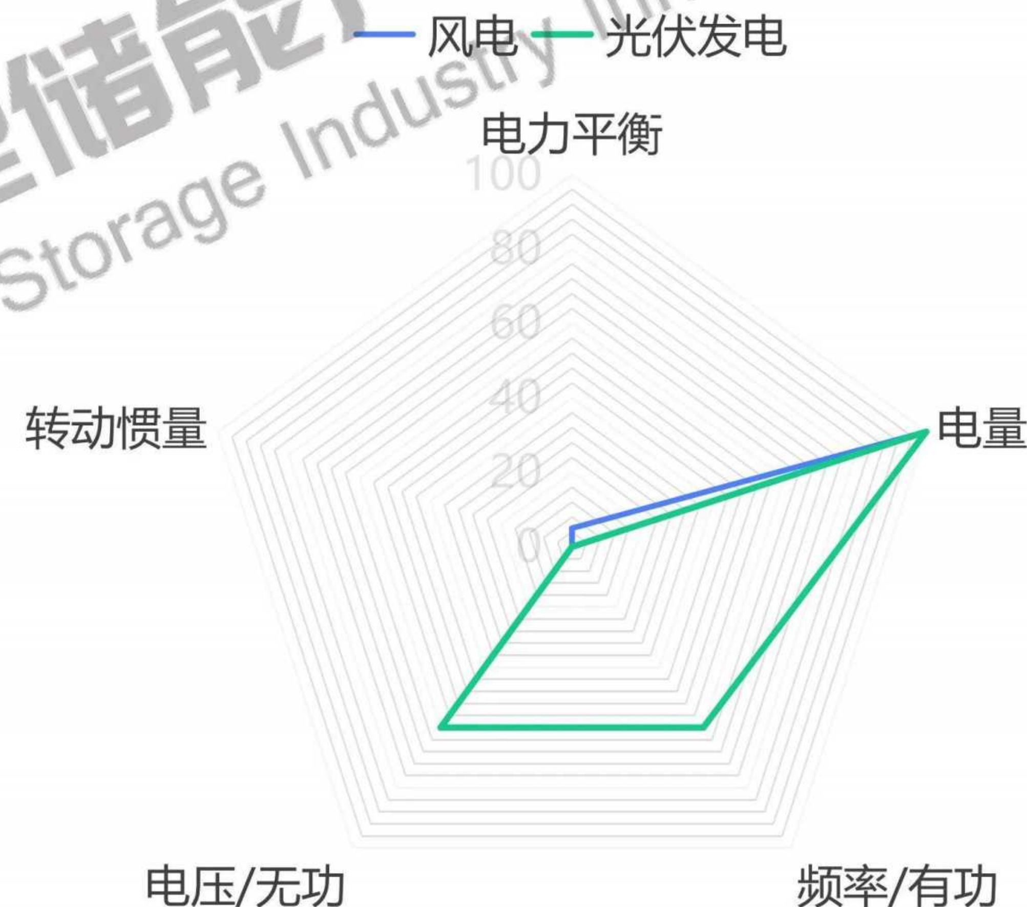
风电光伏发电出力特性图
