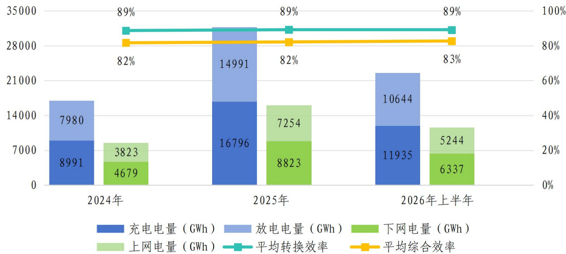
图 3-1 近 3 年电化学储能能效情况
