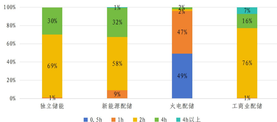
图 1-5 电化学储能典型应用场景储能时长分布情况
