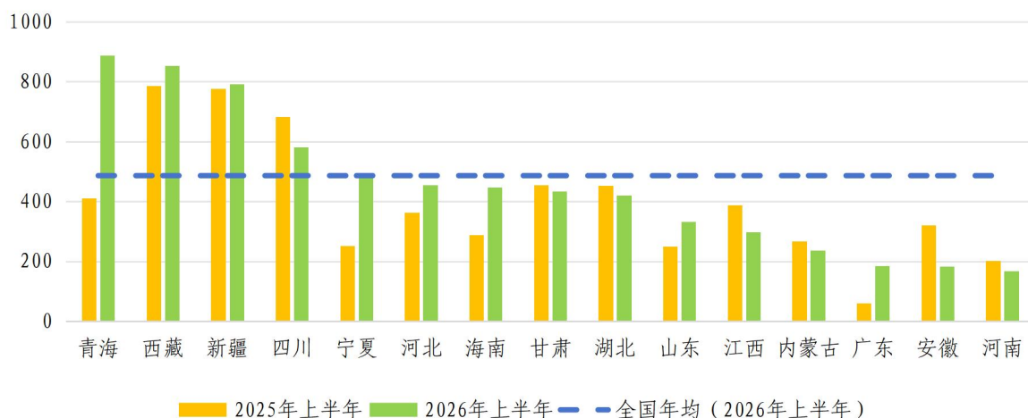
图 2-7 典型区域新能源配储平均利用小时数
