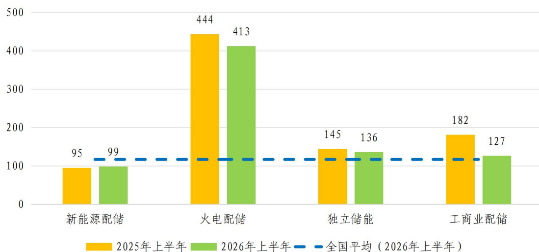
图 2-2 典型应用场景下电化学储能平均等效充放电次数
