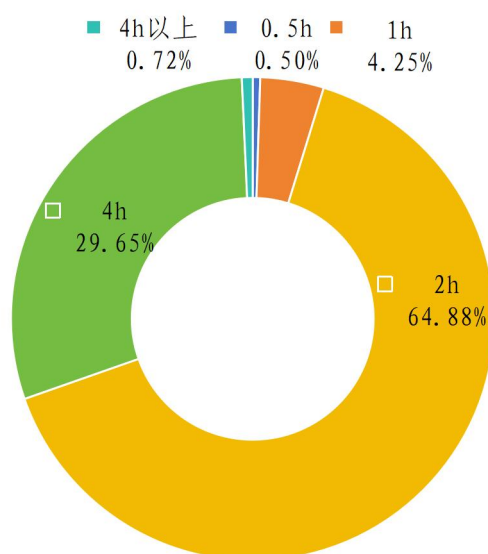
图 1-4 电化学储能储能时长分布情况
