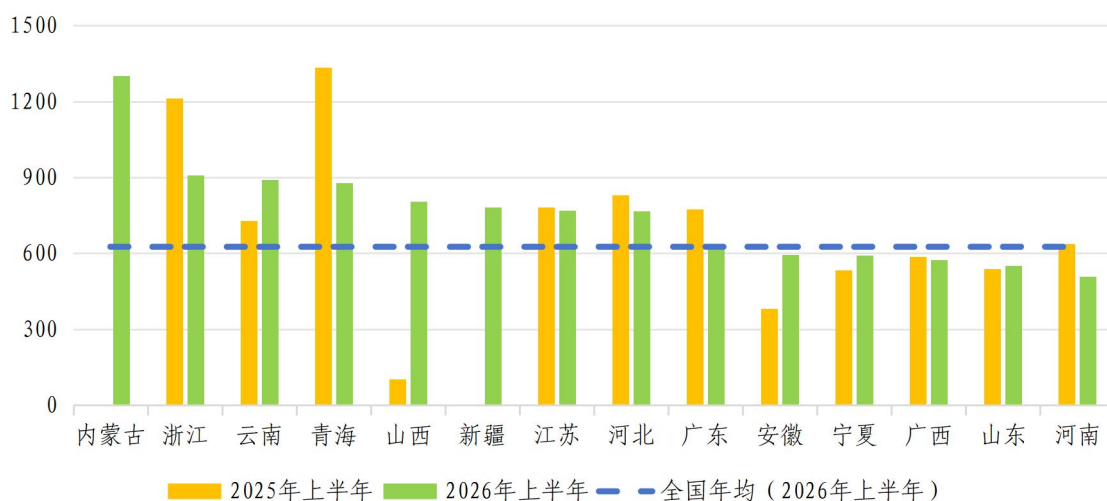
图 2-8 典型区域独立储能平均利用小时数
