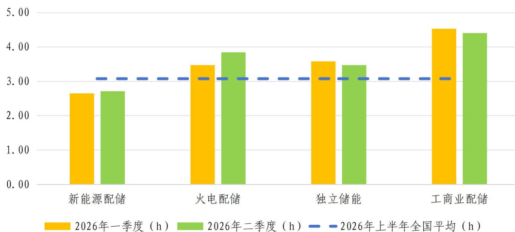
图 2-4 典型应用场景下电化学储能各季度日均利用小时数
