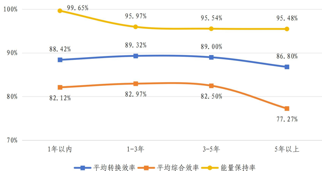
图 3-2 2026 年上半年各投运年限下电化学储能电站能效情况
