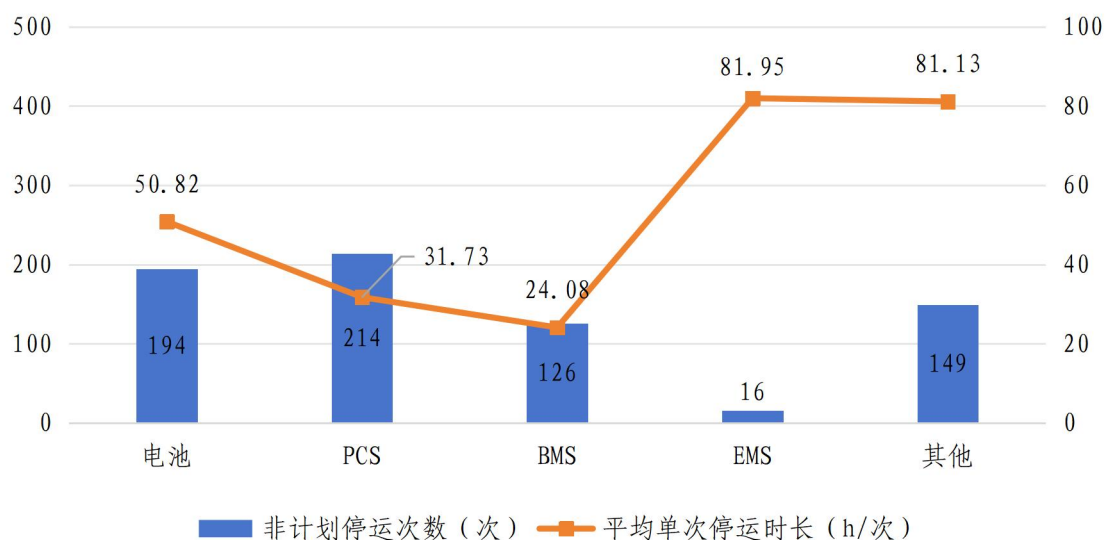
图 4-2 2026 年上半年电化学储能非计划停运情况
