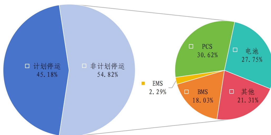
图 4-1 2026 年上半年电化学储能停运次数分布情况
