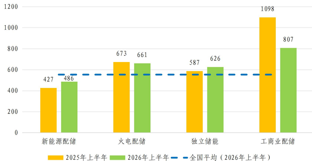
图 2-1 典型应用场景下电化学储能平均利用小时数
