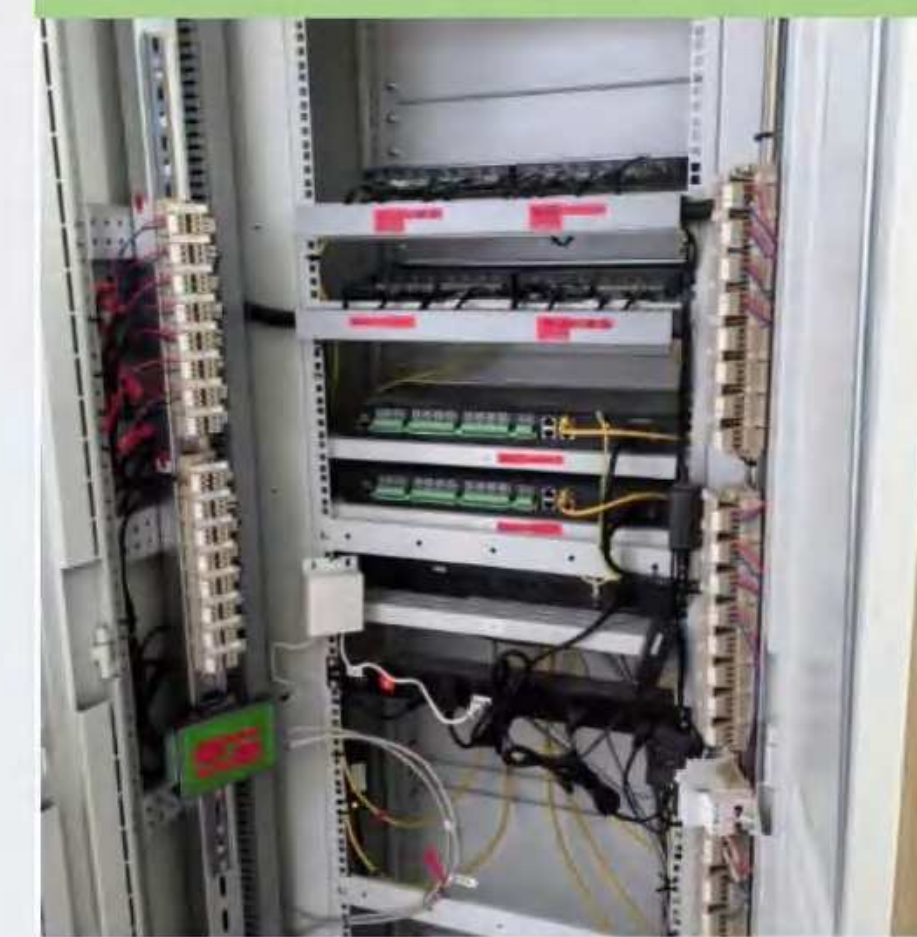
配电柜改造
