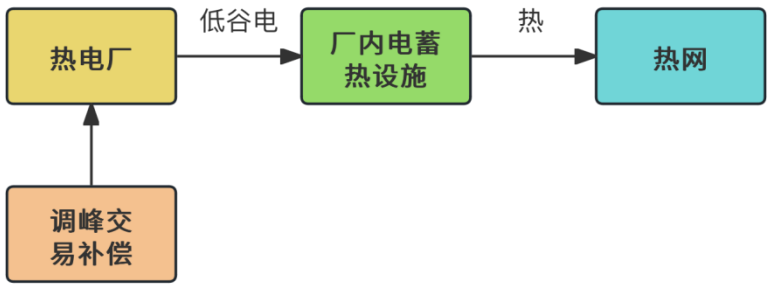
图 5-55：热电厂蓄热改造原理图
