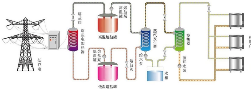
图 5-31：熔盐储热技术流程图
