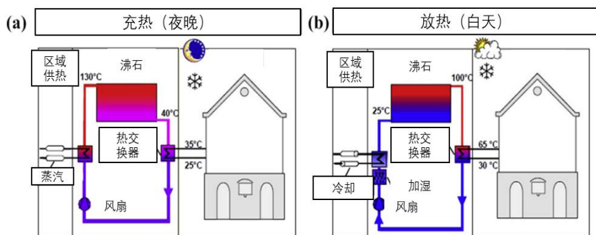
图 2-20：建筑供暖开放式吸附储热系统：(a)供热充电模式；(b)供热放电模式【38】
