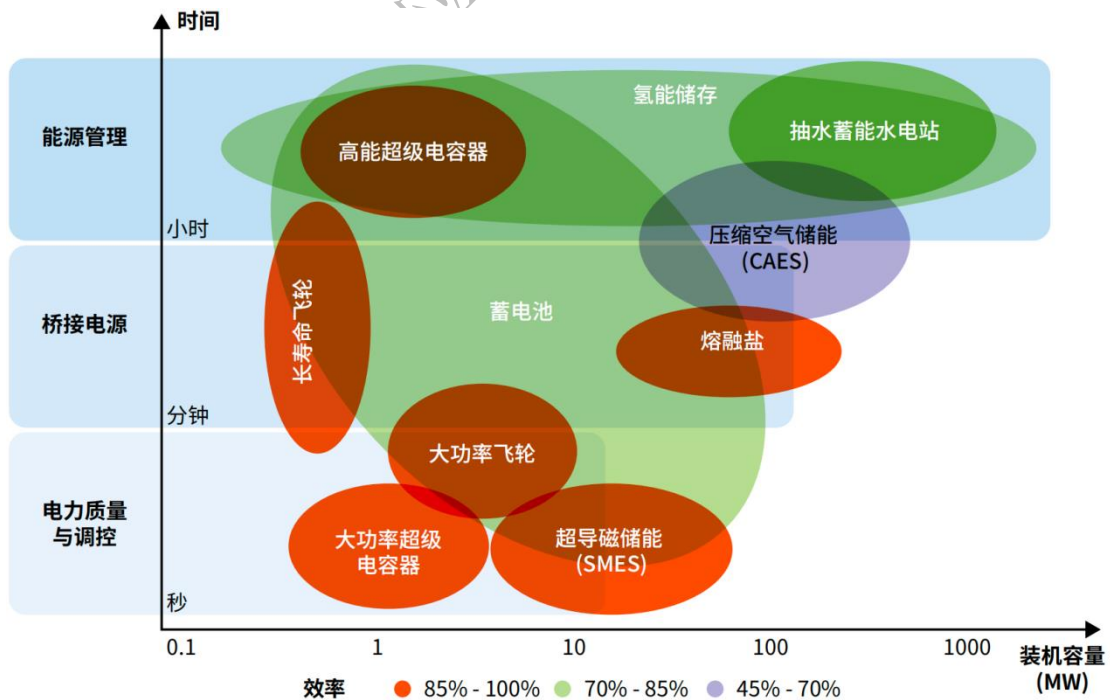
图 5-50：各种储能技术及其在电力系统中的作用【16】
