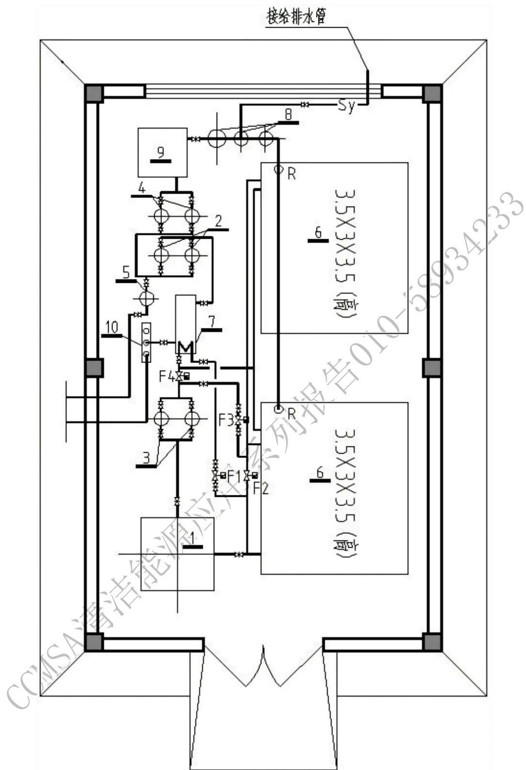
图 6-12：锅炉房设备平面图【89】
