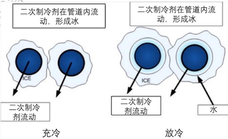
图 2-12：内部盘管冰存储系统的充放电程序【34】
