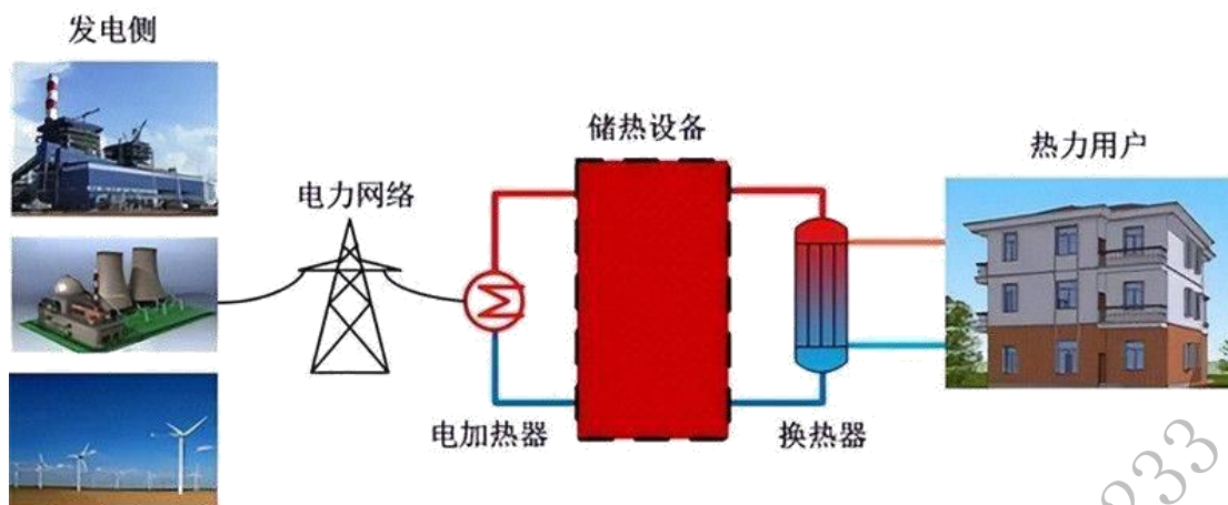
图 5-4：谷电蓄热技术原理示意图
