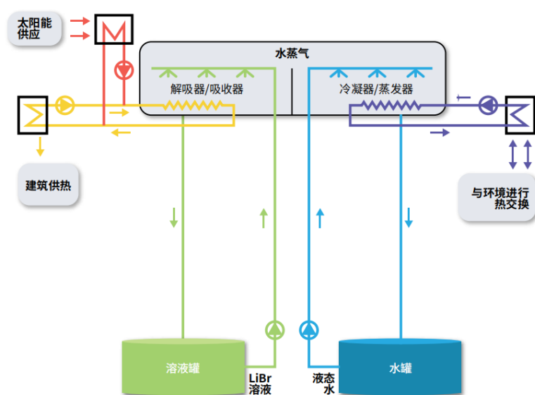
图 2-17：配备分离器反应器的吸收式系统配置【16】
