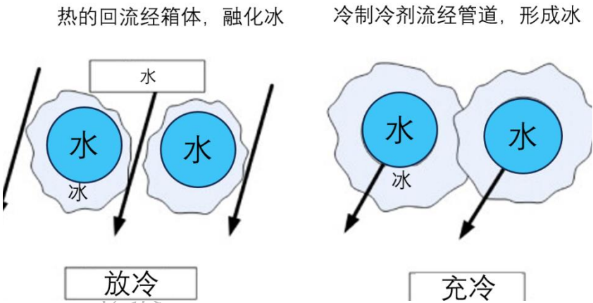
图 2-11：外部融冰储存系统的充放电程序【34】
