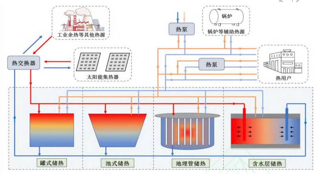
图 5-10：跨季节蓄热储能技术原理示意图【72】
