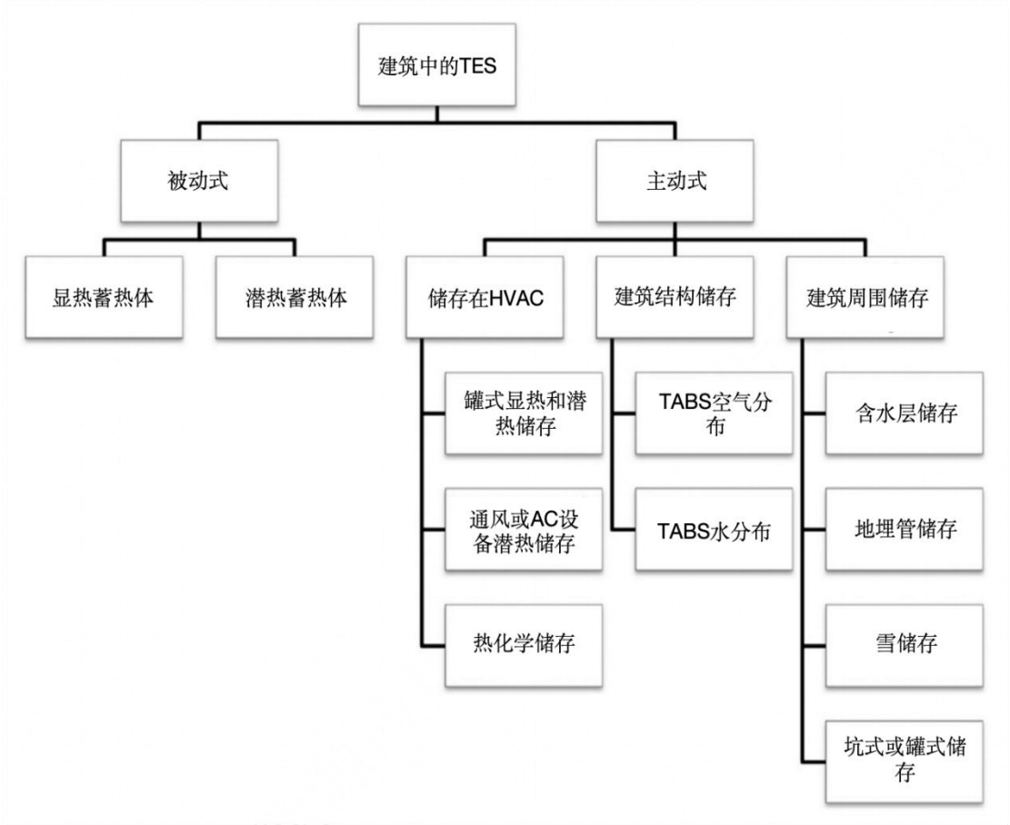
图 5-17: 建筑蓄热储能技术细分【75】
