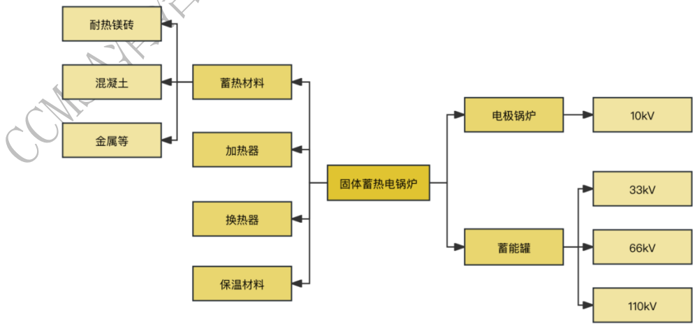
图 6-9：固体蓄热电锅炉产业链图示
