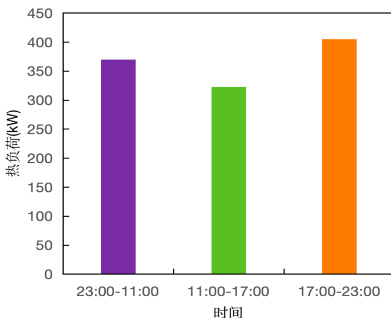
图 6-11: 各时段采暖热负荷汇总【92】
