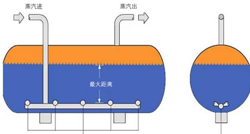
图 2-14: 蒸汽蓄热器示意图 (图片来源: 网络)
