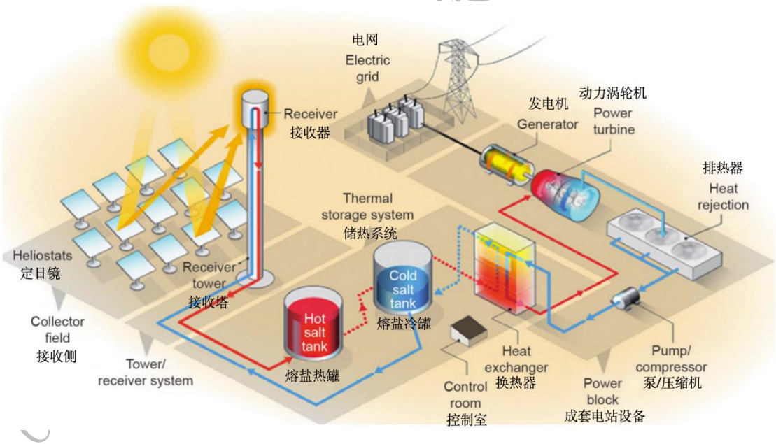
图 5-51：配备熔融硝酸盐直接储热系统的商业化塔式电站【84】
