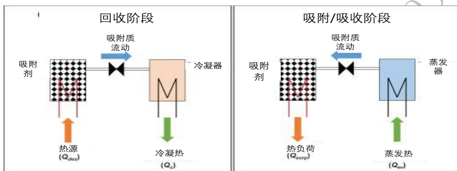
图 2-21：闭式吸附蓄热储能循环：充电和放电阶段【48】
