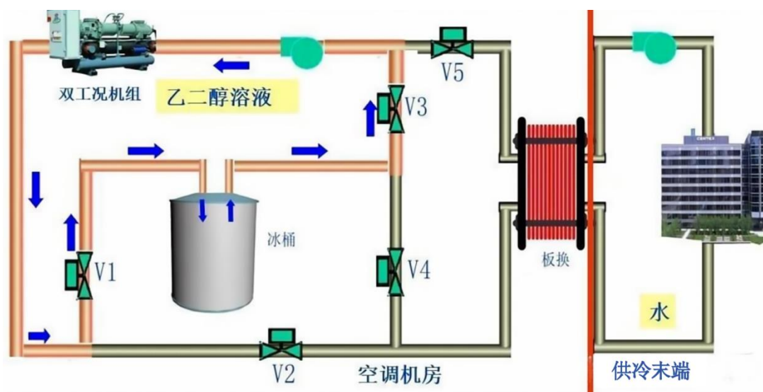
图 5-34：冰蓄冷技术原理流程图【78】
