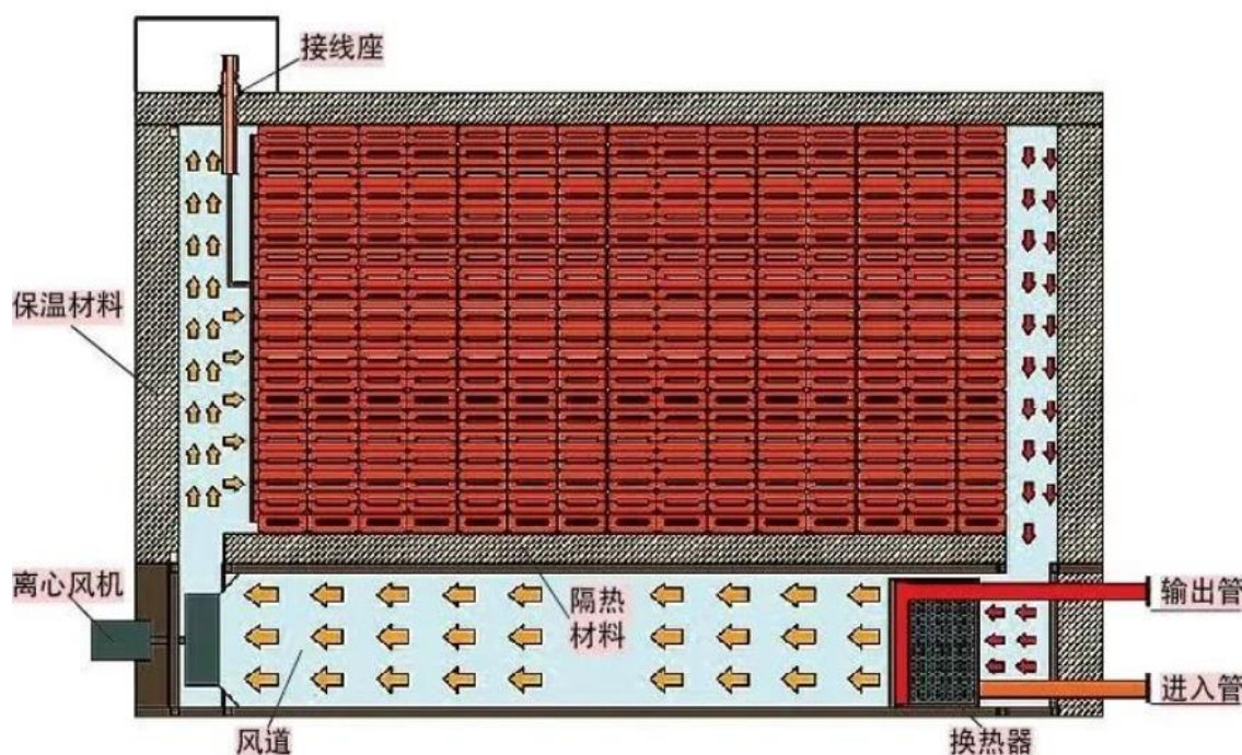
图 5-25：固体蓄热装置工作流程示意图【77】
