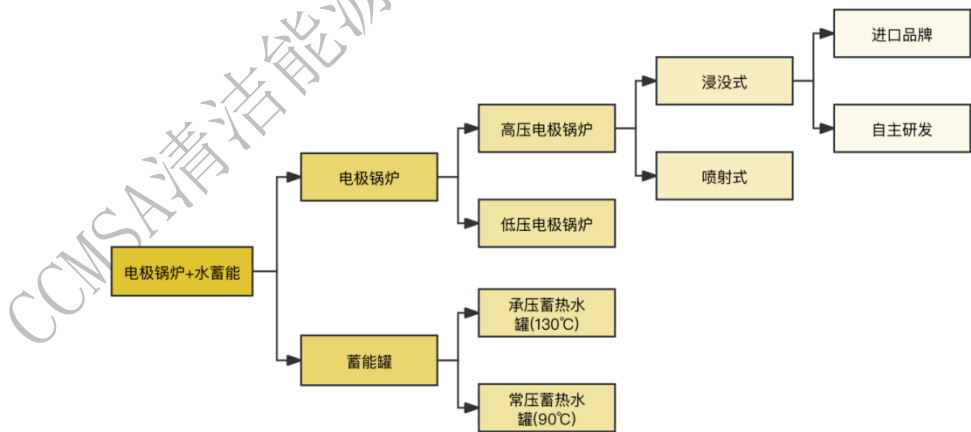
图 6-8：电锅炉+水蓄热储能产业链图示
