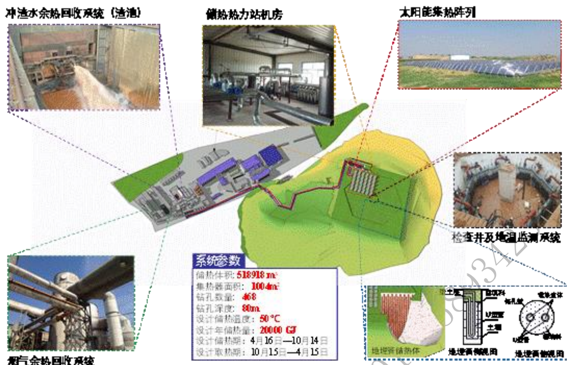
图 5-47:内蒙古赤峰“工业余热+太阳能”跨季节蓄热供暖示范项目
