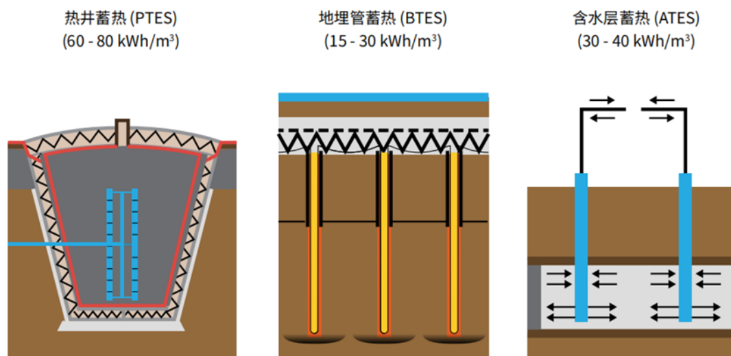
图 2-4：地下蓄热【16】
