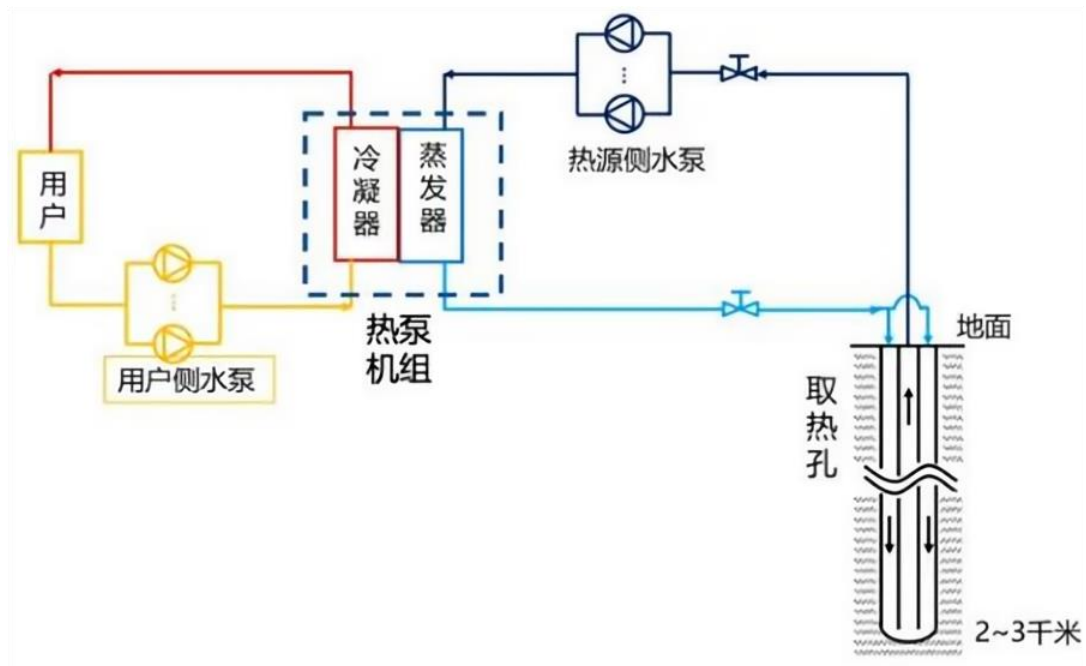
图 5-37：沔西新城地热清洁供热项目工艺流程图
