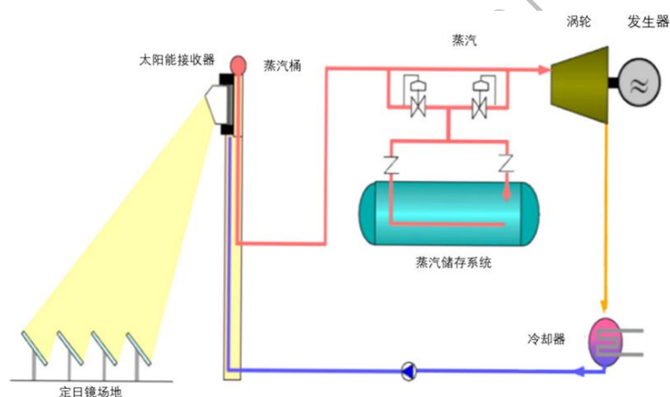
图 2-13：主动式直接蒸汽蓄热储能系统示意图【35】
