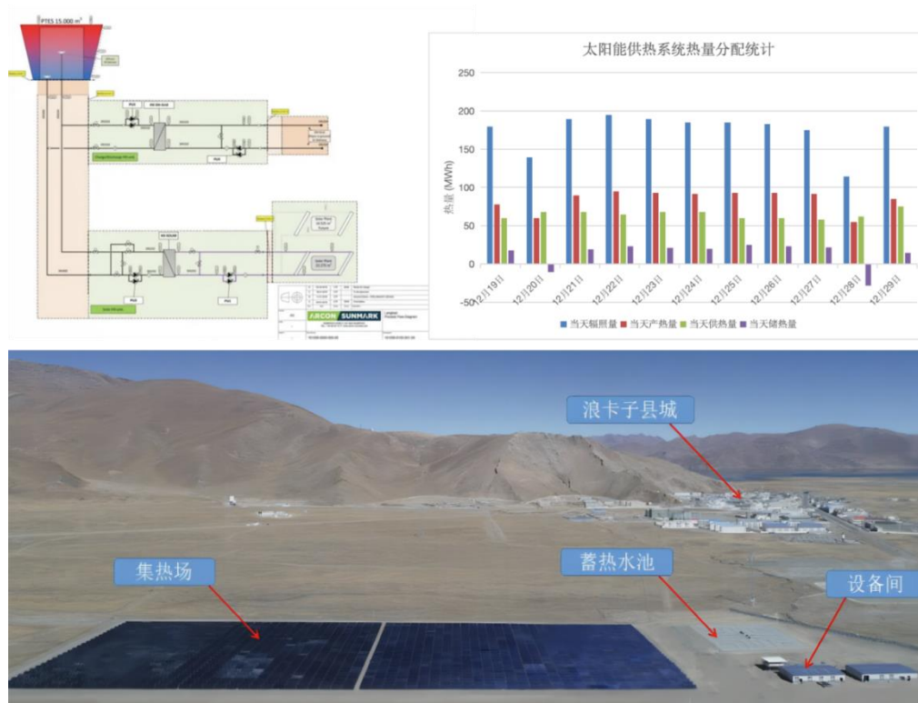
图 5-14: 西藏浪卡子大型太阳能集中供热项目实景图
