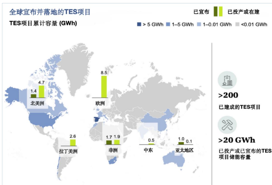
图 5-2：全球年度蓄热储能项目建成数量及储热量统计【67】
