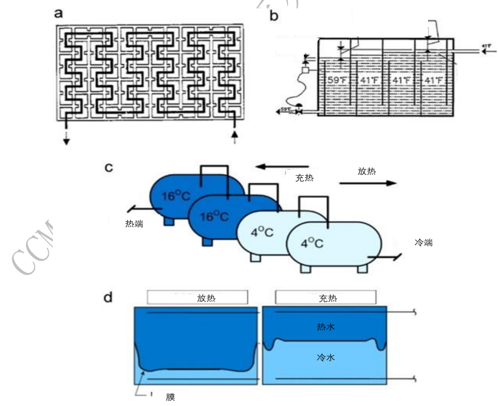
(a) 迷宫式储罐、(b) 挡板储罐、(c) 多蓄水储罐 (d) 隔膜式罐
