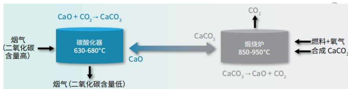
图 2-19: 钙循环过程【16】
