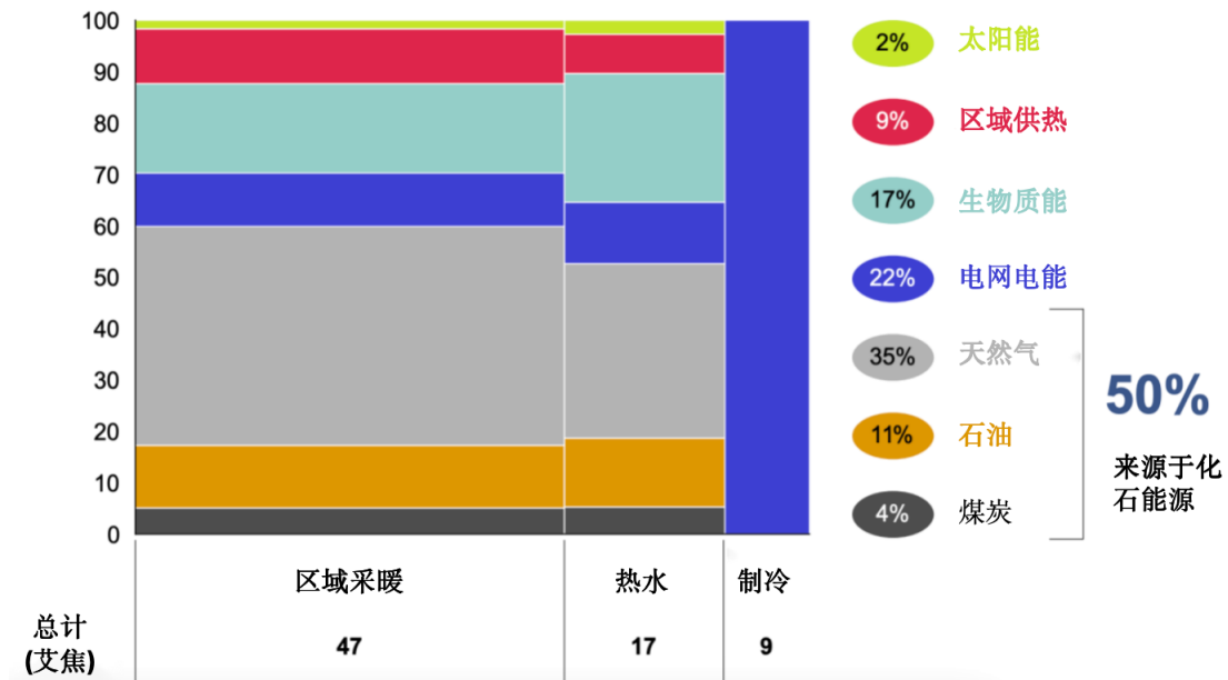
图 5-16: 全球建筑热能能耗占比示意图【67】
