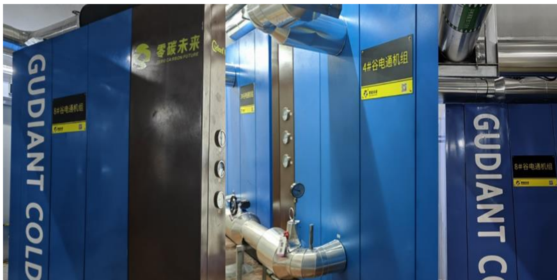
图 5-24：深圳招商局港口大厦 “相变蓄冷+电网谷电” 中央空调蓄冷项目实景图
