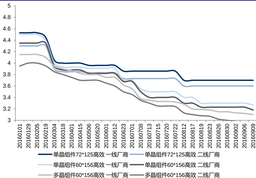
图 4：光伏组件价格趋势图（单位：元/瓦）
