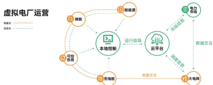
图2：虚拟电厂参与需求侧响应
